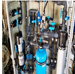
Úprava vody
